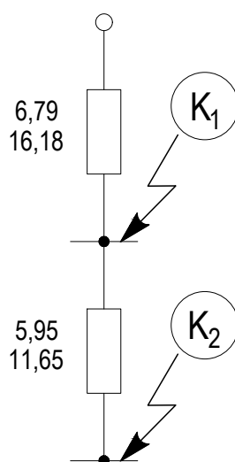
Рисунок 8.2 – Схема замещения защищаемого трансформатора и результаты расчета токов КЗ
