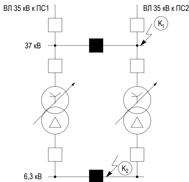
Рисунок 8.1 – Поясняющая схема и схема замещения защищаемого трансформатора
